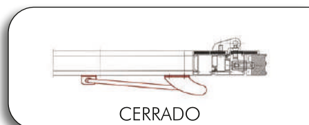
Ref: RETE300-3 (Para hojas mayores de 450 mm)
