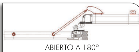
Ref: RETE300-3 (Para hojas mayores de 450 mm)
