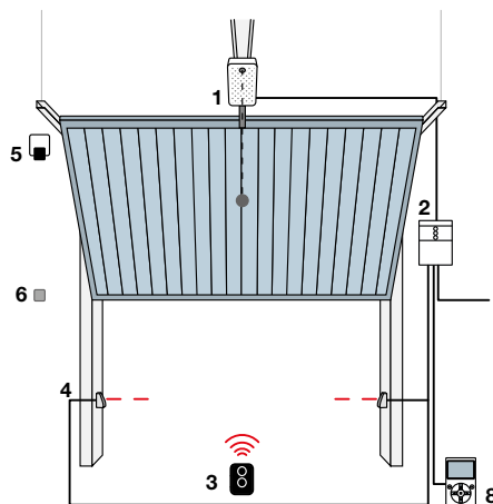
Basculante no desbordante
