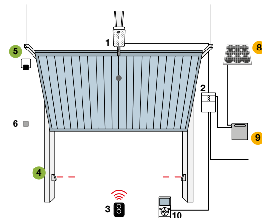
Basculante no desbordante
