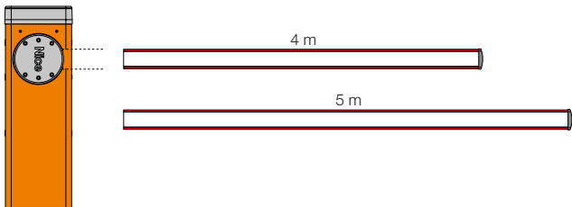
M5BAR Con mástil de 4 m Preinstalación para: goma de protección, luces de señal, bastidor (1 ud.),
