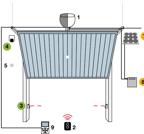
Basculante no desbordante
