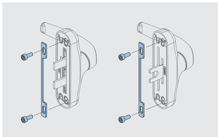
Sistema de fijación CLASSIC 0710 · 0720 · 0760 · P0760
