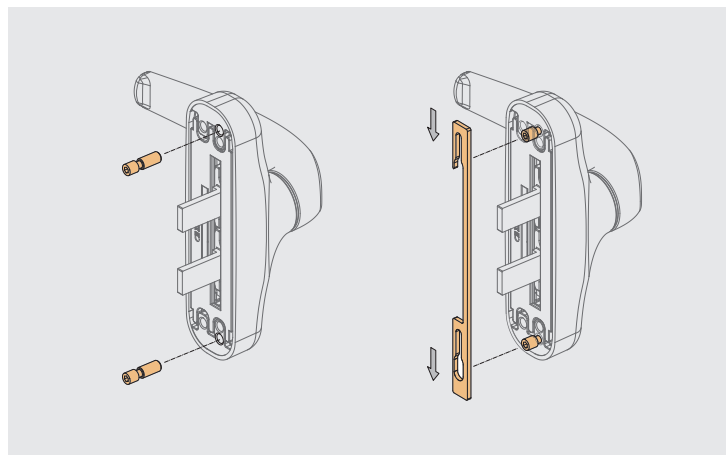
Sistema de fijación FAST 0710 · 0720
