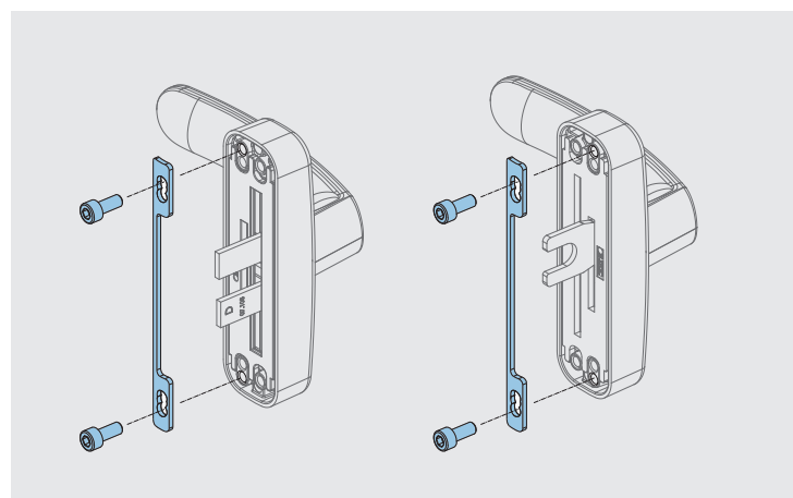
Sistema de fijación CLASSIC A0790 · A0791 · A0794 · P0794
