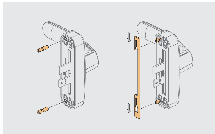
Sistema de fijación FAST A0790 · A0791 · A0794 · P0794
