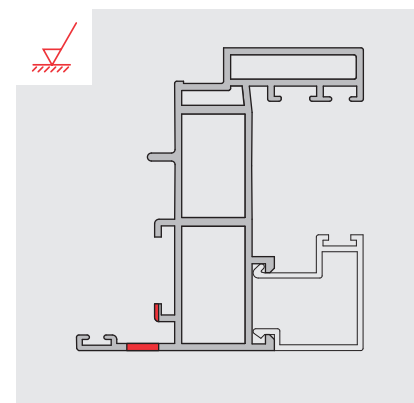
sección de perfil A-A
