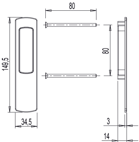
Dimensiones tirador
